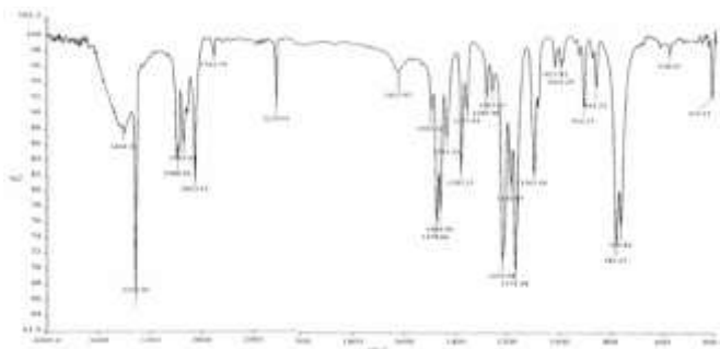
1-Rasm. Bisbuteronitrildiaminning IQ-spektri
